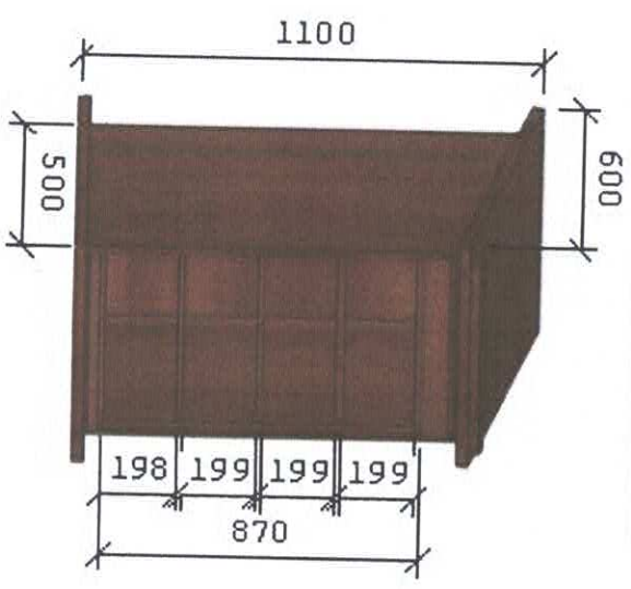
VISTA LATERAL
