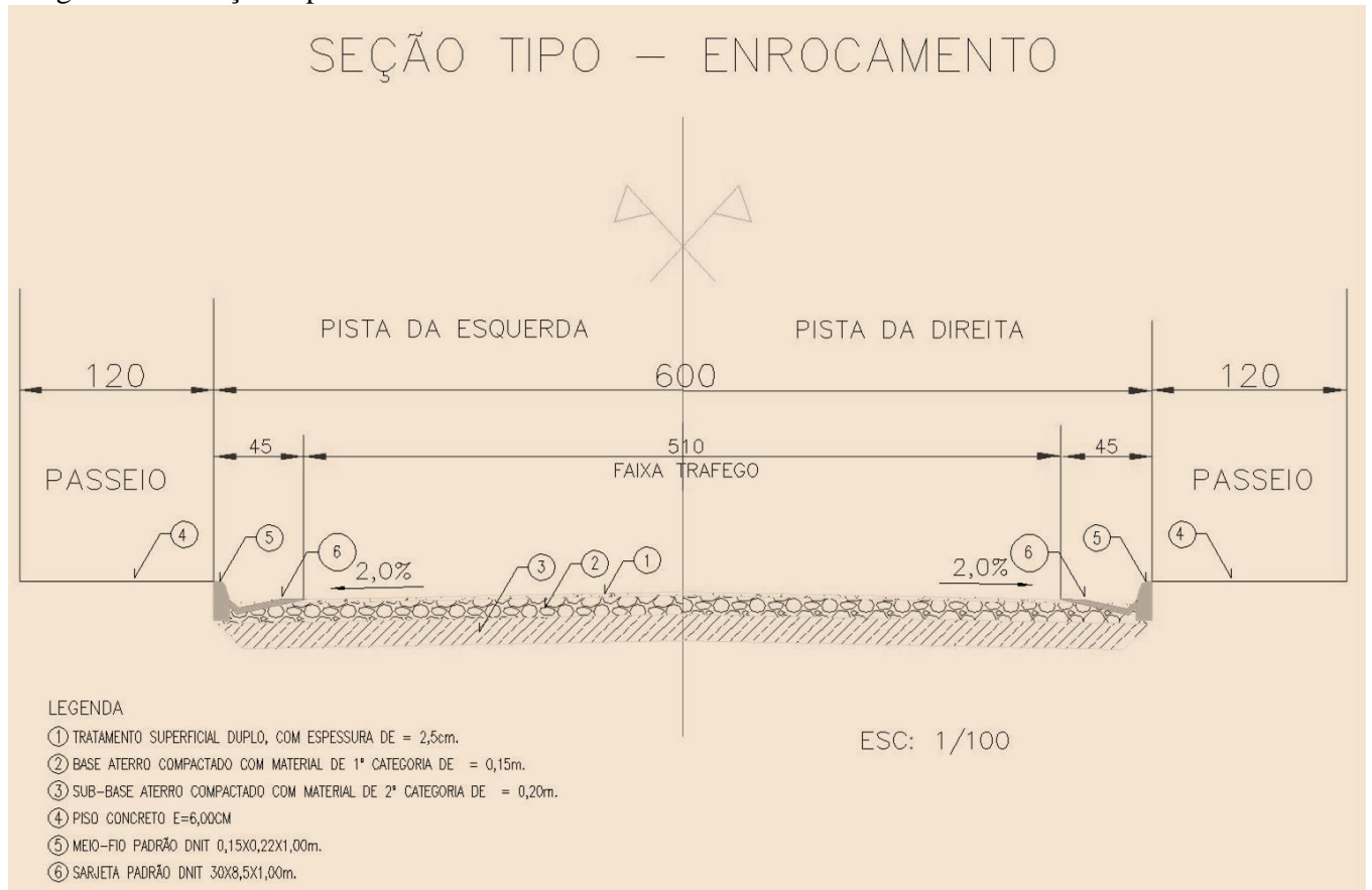
Imagem 003 - Seção Tipo
